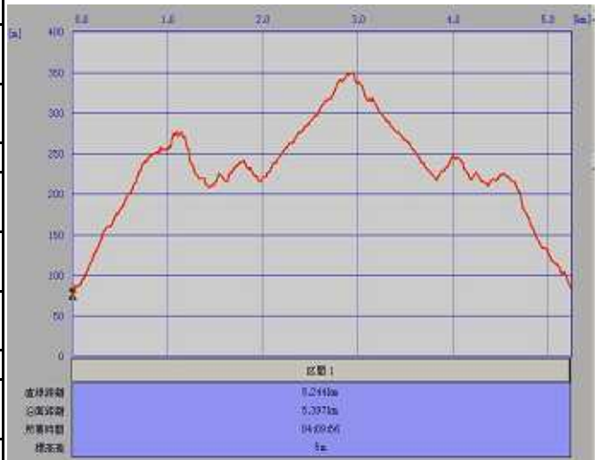
* 行程グラフ
